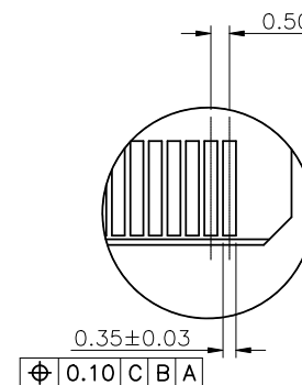
DETAIL : D SCALE 4 : 1
