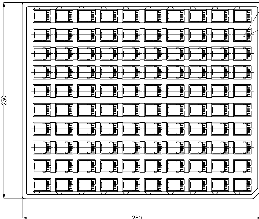
产品放入盘内，端子焊脚朝右，100 PCS/TRAY
