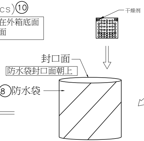
④ 10盘产品入防水袋示意图
