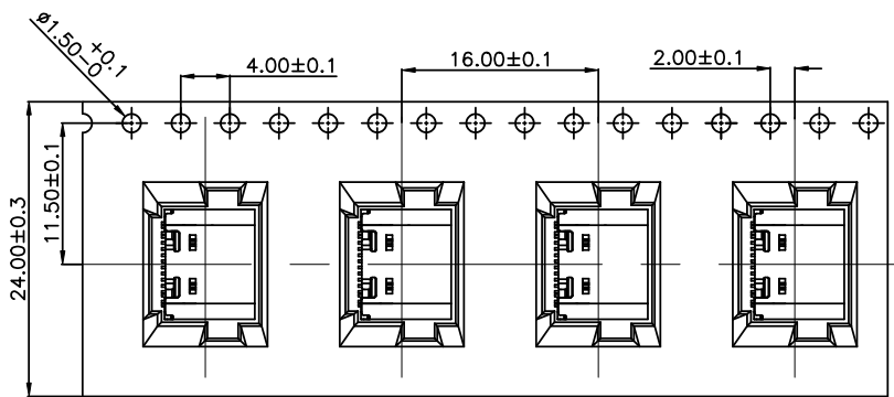
② 产品入载带示意图
